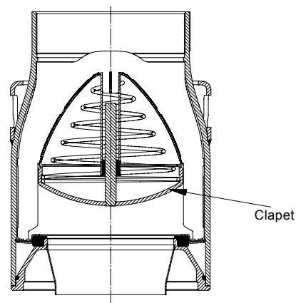
Fig. 5 Clapet anti-retour
